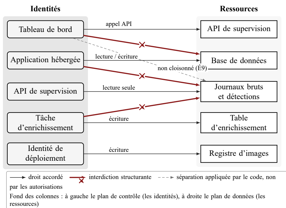
FIG. 16. Plan d'identité : droits accordés et interdictions structurantes (cinq identités). Ni l'application hébergée ni la tâche d'enrichissement ne peuvent écrire sur les preuves (scénario SO16, test T11); le tableau de bord passe par l'API de supervision, mais son identité conserve un droit de lecture sur l'entrepôt — c'est l'écart É9.
