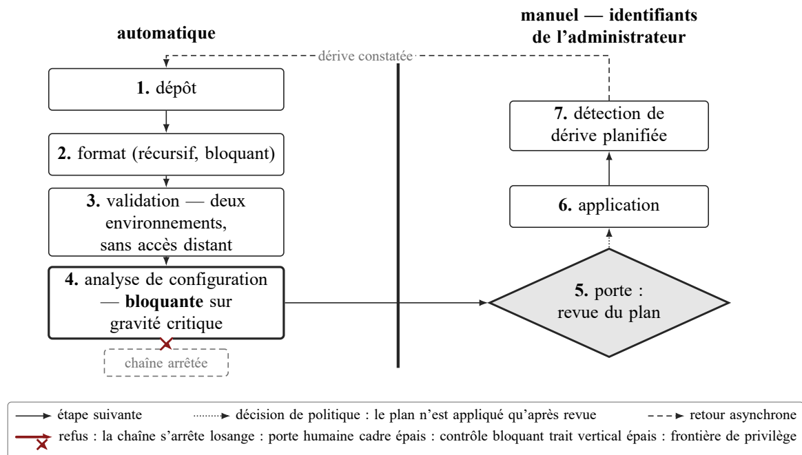
FIG. 20. Chaîne de provisionnement de l'infrastructure : la frontière automatique/manuel est un choix de privilège , non un degré d'achèvement — la partie automatisée n'a, par construction, aucun accès au fournisseur cloud.
